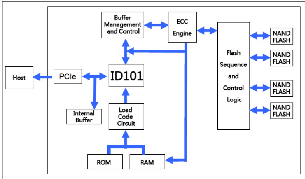
Figure 2: InnoDisk Mini PCIeDOM D150 Block Diagram
